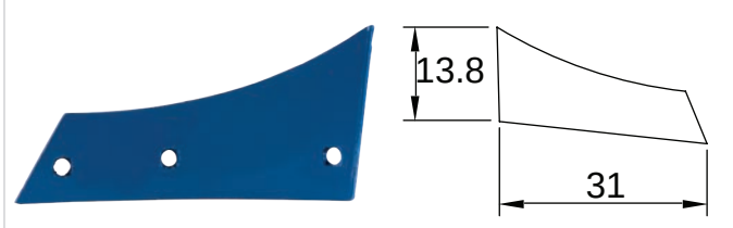
K-231 Ünlü Kulak Ön Parçaları
