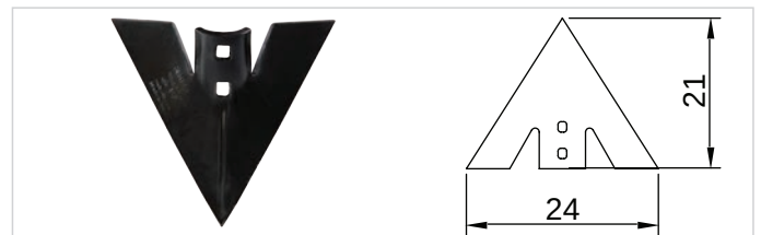
K-205 BirleşimBOR 7 mm 24 cm Kultivatör Bıçağı
