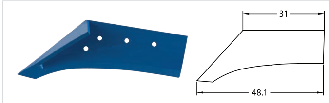
B-116 Ünlü 10 No Bıçak (Üçgen Parça Kaynaklı)
