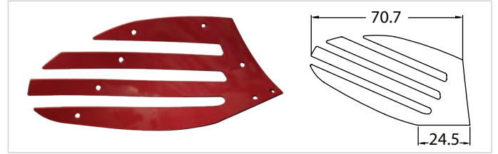
K-301 Ünlü - Izgara Ayna 14 No
