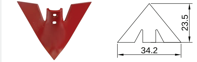
K-202 Krone Kültivatör Bıçağı 8 mm
