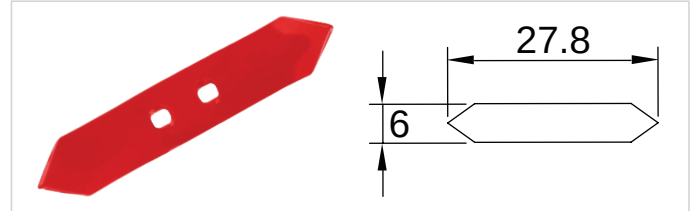
K-248 Kültivatör için Yılandili 10 mm
