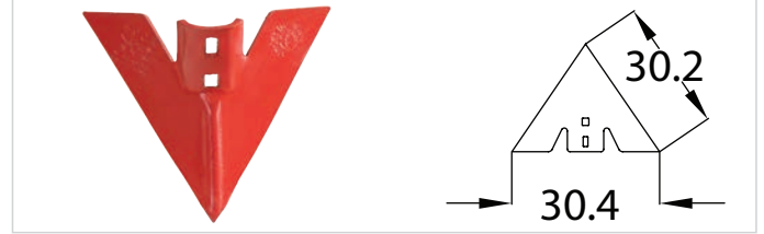
1112 BirleşimBOR 7 mm - 30 cm Kultivatör Bıçağı
