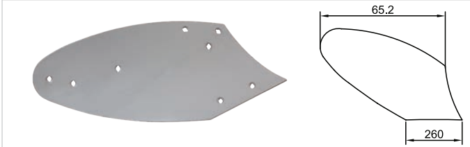
K-244 Alpler - Aydın 11 No Kulakları (AYNA)
