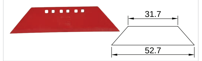
B-122 Turun 14 inç - 6 Delik
