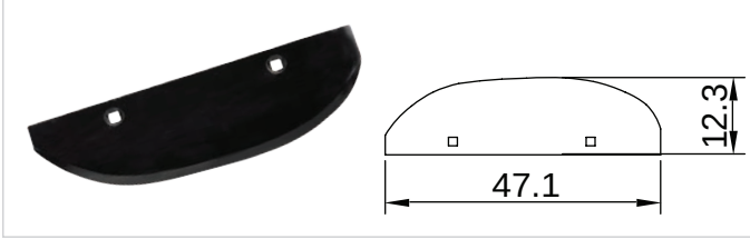
K-255 Pancar Söküm Bıçağı HARMAK
