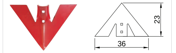
K-203 Parmiter Kültivatör Bıçağı 8 mm
