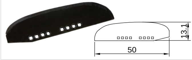
K-263 Pancar Söküm Bıçağı ALTINÖRS (8 Delikli)
