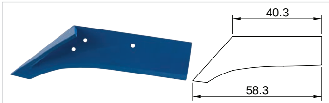
B-136 Ünlü 14 - 16 No Bıçak (Üçgen Parça Kaynaklı)
