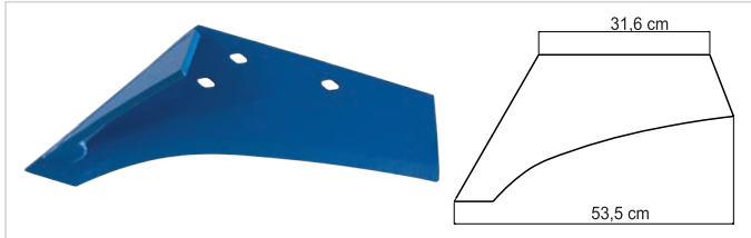
B-101 Alpler - Aydın 14 No
