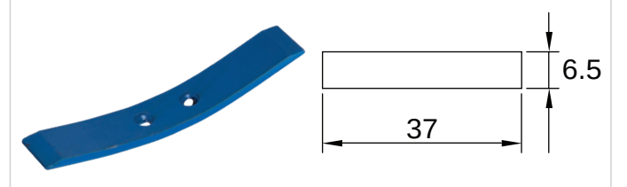
K-265 Esener-Matris Çizel Pulluk Bıçağı (Anız Patlatan) 5mm / 37mm / 12mm
