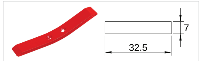
K-269 Çizel Pulluk Bıçağı (Anız Patlatan) 70mm / 32mm / 14mm
