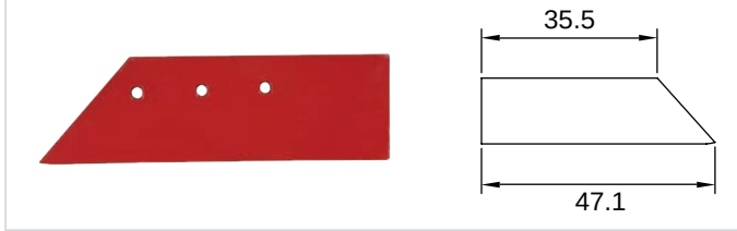
B-131 Ünlü Bıçak Gövdesi 18 No
