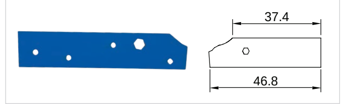
T-125 Ünlü 9 No Taban Demiri - Uzun
