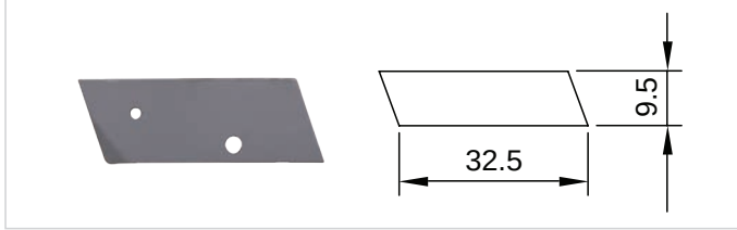
T-122 Alpler - Aydın 10 - 12 - 14 Taban Demiri - Kısa Yeni
