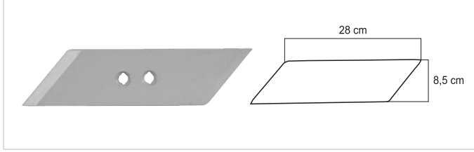
B-138 Alpler - Aydın Ön Parça
