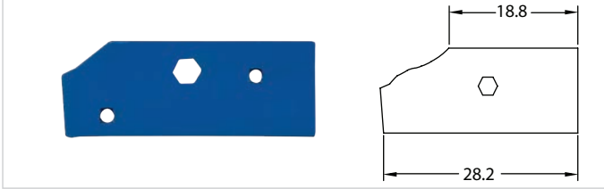
T-124 Ünlü 9 No Taban Demiri - Kısa
