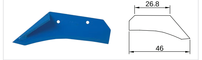
B-144 Ünlü 8 No Bıçak Geniş Ara (Üçgen Parça Kaynaklı)
