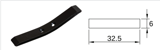
K-208 Çizel Pulluk Bıçağı (Anız Patlatan) 60mm / 32mm / 12mm
