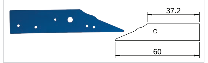
T-113 Ünlü Taban Demiri - Uzun
