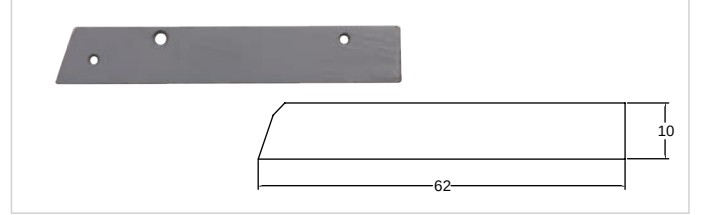
T-119 Alpler - Aydın 8 No Taban Demiri - Uzun
