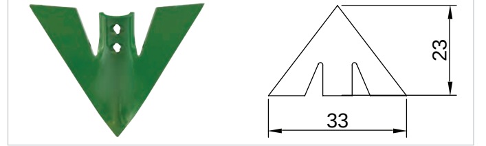
K-241 Ekermak ve Yıldırım 2004 Kültivatör Bıçağı 8 mm
