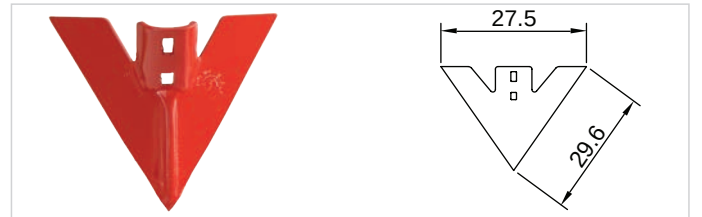
1107 BirleşimBOR 7 mm - 27 cm Kültivatör Bıçağı
