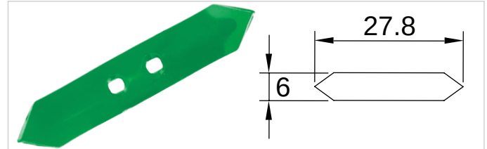
K-250 Kültivatör için Yılandili 14 mm
