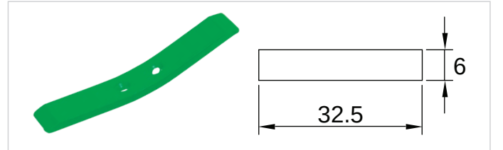
K-266 Çizel Pulluk Bıçağı (Anız Patlatan) 60mm / 32mm / 14mm
