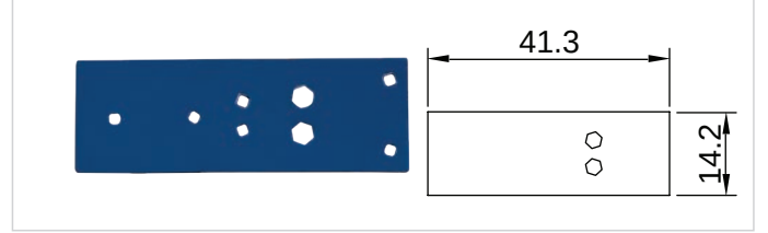
T-127 Ünlü Taban Demiri Gövdesi
