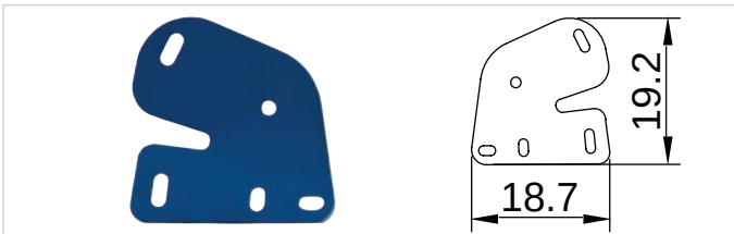
B-136 Ünlü Toprak Devirme Gövdesi
