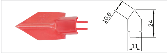
1103 Birleşim PlatinBOR 8 mm Çizel Pulluk Bıçağı
