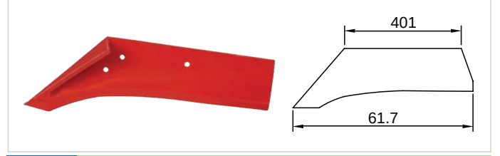
B-123 Alpler - 6 Soklu Bıçak
