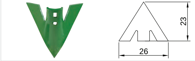
K-204 Zirai Donatım Kurumu Kültivatör Bıçağı 8 mm
