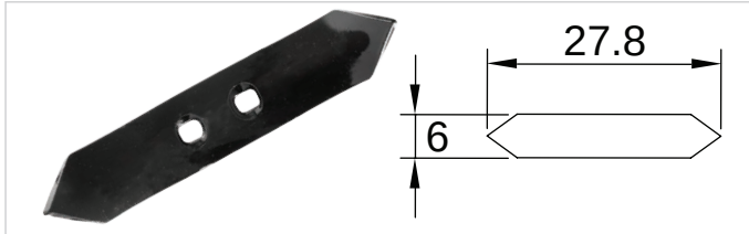
K-249 Kültivatör için Yılandili 12 mm
