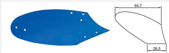
K-220 Alpler - Aydın 14 No Kulakları (AYNA)
