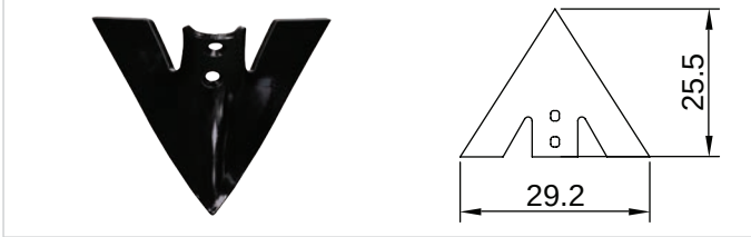
K-225 BirleşimBOR 7 mm - 29 cm Kültivatör Bıçağı
