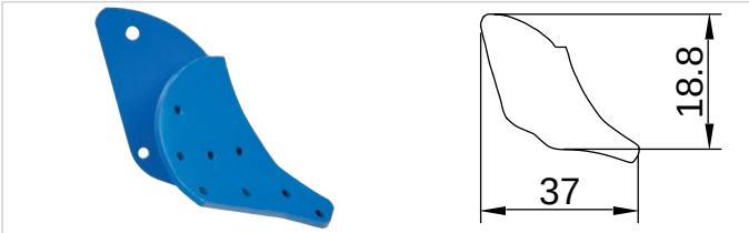
A-108 Ünlü 9 No Ana (Payanda)
