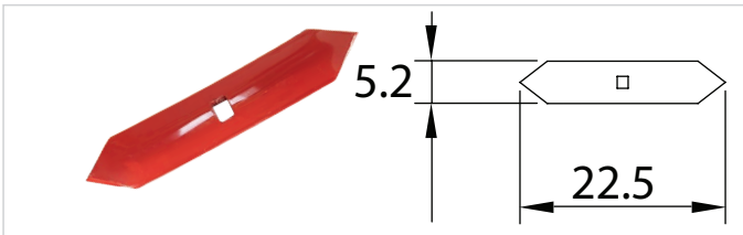
K-226 Birleşim Yaykürüm (Aysan) Bıçakları 7 mm (Yılandili)
