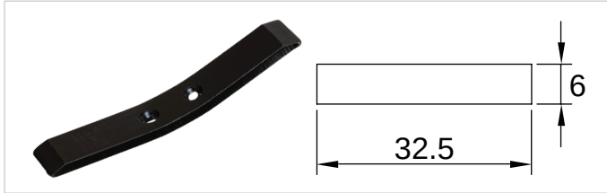
K-265 Çizel Pulluk Bıçağı (Anız Patlatan) 60mm / 37mm / 12mm
