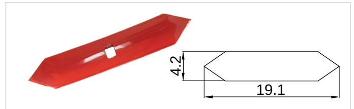
K-226 Birleşim Yaykürüm (Aysan) Bıçakları 7 mm (Yılandili)
