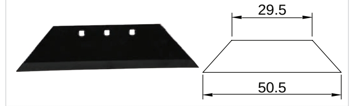
B-118 Turun 11 - 13 inç - 12 mm
