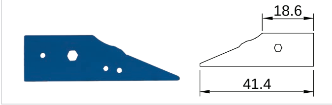
T-112 Ünlü Taban Demiri - Kısa
