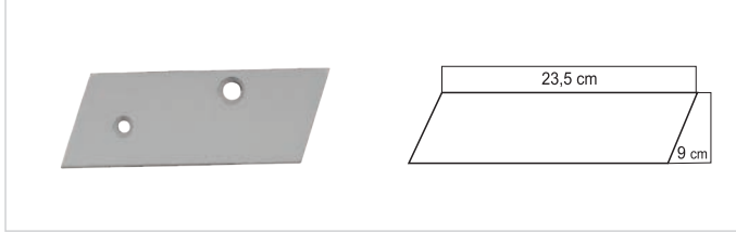
T-107 Alpler - Aydın 10 - 12 - 14 Taban Demiri - Kısa
