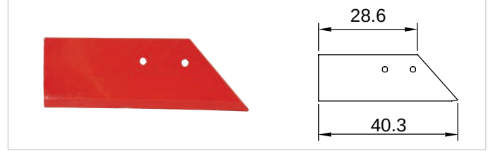
B-129 Ünlü Bıçak Gövdesi 10 - 12 - 13 No (Sağ - Sol)
