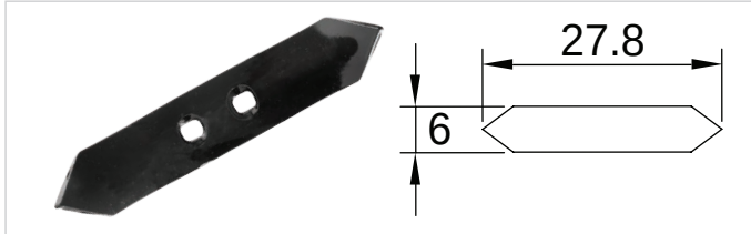
K-247 Kültivatör için Yılandili 8 mm
