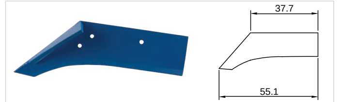
B-125 Ünlü 12 No Bıçak (Üçgen Parça Kaynaklı)
