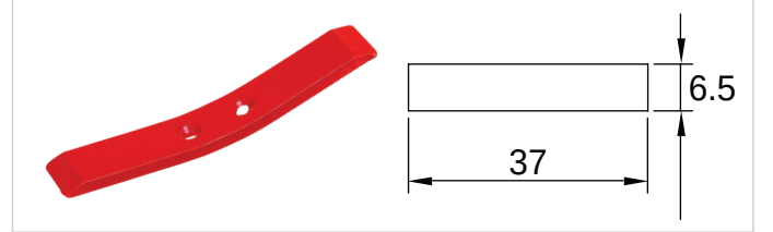
K-224 Döküm Bacak Çizel Pulluklar için Kültivatör Bıçağı 8 mm
