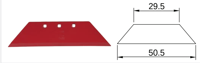
B-108 Turun 11 - 13 inç - 3 Delik
