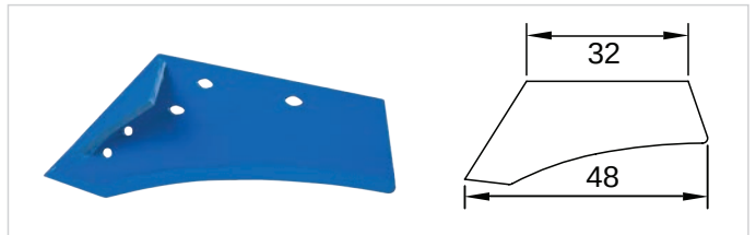
B-140 Alpler - Aydın 14 No Parçalı Arka Bıçak
