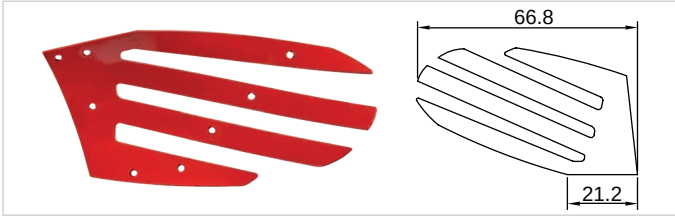
K-300 Ünlü - Izgara Ayna 12 No
