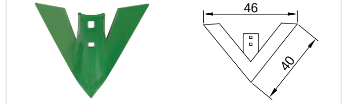
K-202 Krone Kültivatör Bıçağı 10 mm
