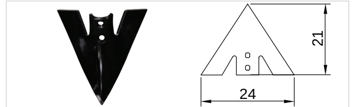
K-239 BirleşimBOR 8 mm 24 cm Kültivatör Bıçağı
