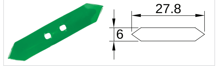
K-207 Kültivatör için Yılandili 7 mm
