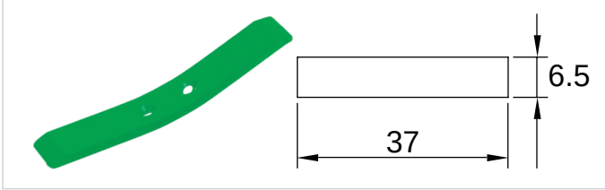
K-240 Döküm Bacak Çizel Pulluklar için Kültivatör Bıçağı 10 mm
