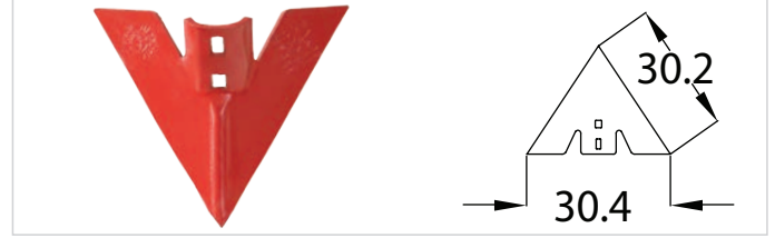
1113 BirleşimBOR 10 mm - 30 cm Kultivatör Bıçağı
