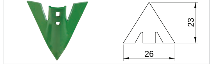
K-212 Zirai Donatım Kurumu Kültivatör Bıçağı 10 mm
