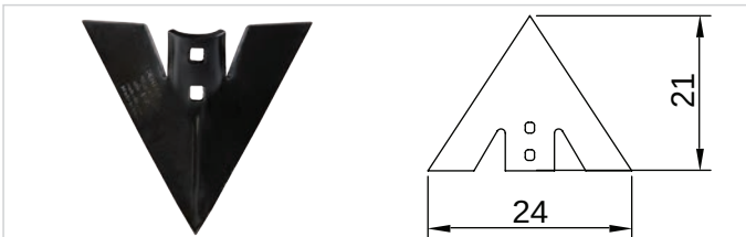
K-239 BirleşimBOR 8 mm 24 cm Kultivatör Bıçağı
