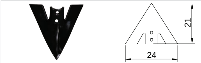
K-205 BirleşimBOR 7 mm 24 cm Kültivatör Bıçağı
