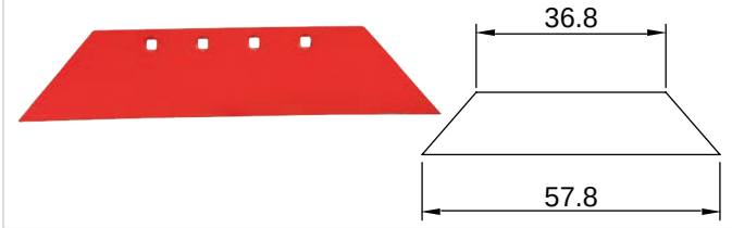
B-126 Turun 16 inç - 4 Delik
