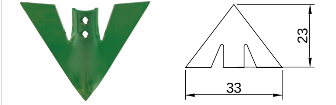
K-219 Ekermak ve Yıldırım 2004 Kültivatör Bıçağı 10 mm
